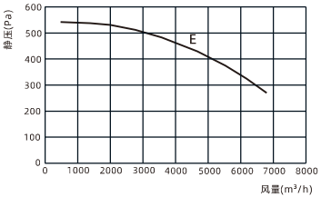
QFA-D6000P (-Y) 性能曲线图
