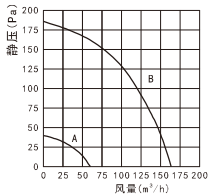
A: DGT10-24TP-D最弱档 B: DGT10-24TP-D最强档
