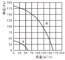
A: DGT10-24TP最弱档 B: DGT10-24TP最强档
