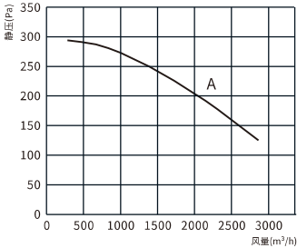
QFA-D2500P (-Y) 性能曲线图
