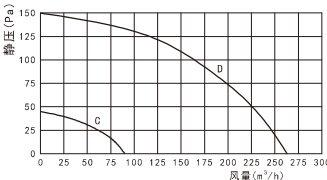
C: DGT15-33TP-D最弱档 D: DGT15-33TP-D最强档
