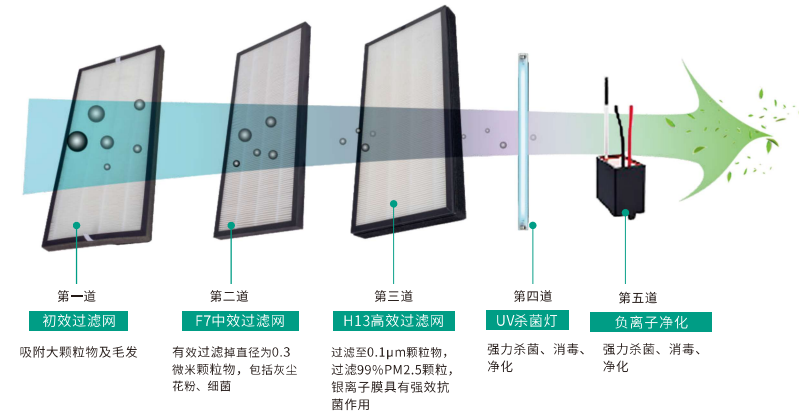
产品过滤杀毒示意图
