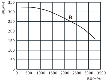
QFA-D3000P (-Y) 性能曲线图
