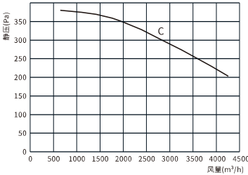
QFA-D4000P (-Y) 性能曲线图
