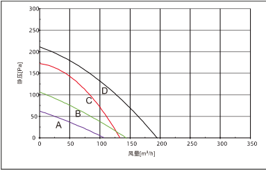
DST10-150P DST10-150P-Y 静压-风量性能曲线图
