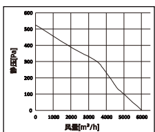
DUT-D6000性能曲线图
