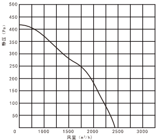
QFA-D2500S、QFA-D2500S-Y静压-风量性能曲线
