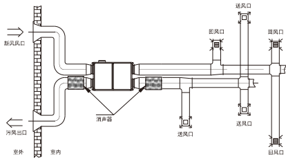
俯视-安装示意图
