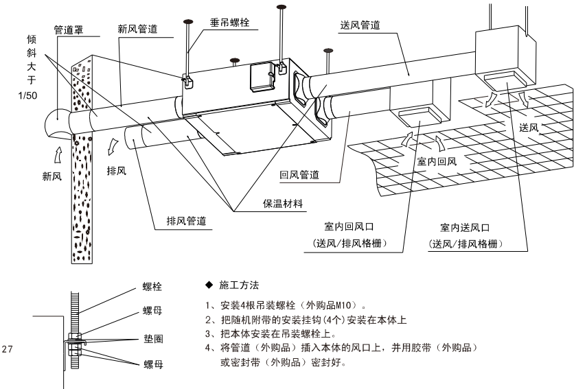
安装示意
