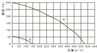
G: DGT20-45TP最弱档 H: DGT20-45TP最强档
