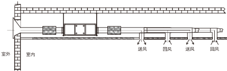
侧视-安装示意图
