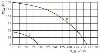
C: DGT15-33TP最弱档 D: DGT15-33TP最强档
