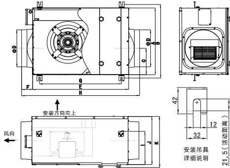
图示所属机型: DGT25-56H/DGT25-66H/DGT25-76H
