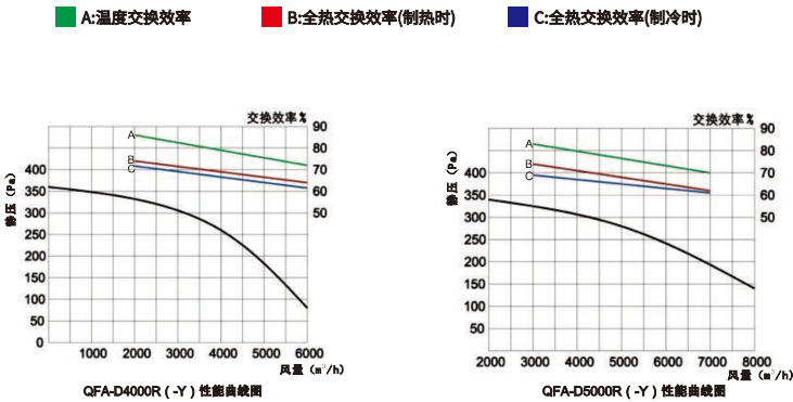
风量4000m³/h–10000m³/h 性能曲线图
