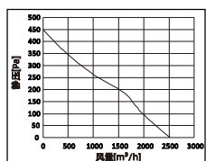
DUT-D2500性能曲线图
