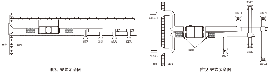
侧视-安装示意图
