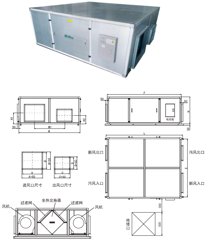
风量4000m³/h–10000m³/h 外形尺寸图
