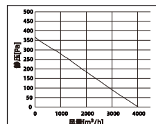
DUT-D4000性能曲线图
