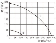
E: DGT15-35TP最弱档 F: DGT15-35TP最强档
