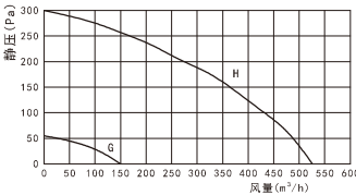
G: DGT20-45TP-D最弱档 H: DGT20-45TP-D最强档
