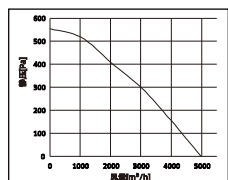
DUT-D5000性能曲线图
