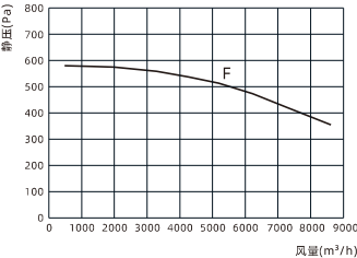
QFA-D8000P (-Y) 性能曲线图
