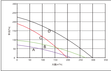
DST15-250P DST15-250P-Y 静压-风量性能曲线图
