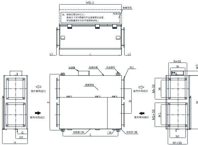
产品尺寸
