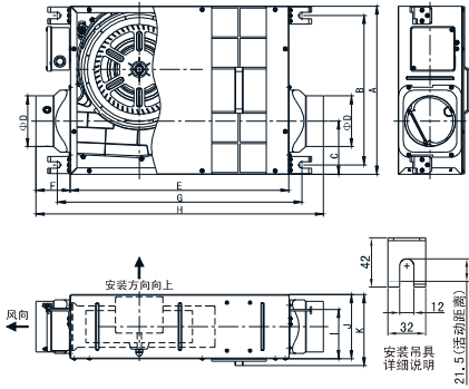
图示所属机型: DGT10-24H(-Y)/DGT15-34H(-Y)/ DGT15-45H(-Y)/DGT15-55H/DGT20-56H/DGT20-56J
