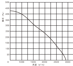
QFA-D3000S、QFA-D3000S-Y静压-风量性能曲线
