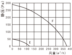
E: DGT15-35TP-D最弱档 F: DGT15-35TP-D最强档
