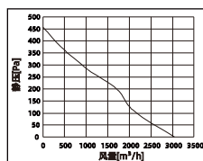
DUT-D3000性能曲线图
