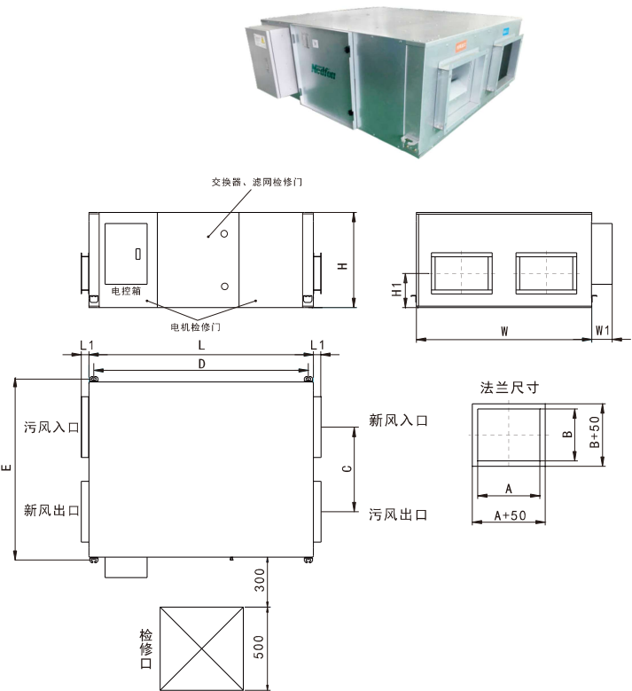
风量2500m³/h-3000m³/h 外形尺寸图
